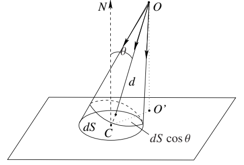
Fig. 4. Illuminance on unit area dS
